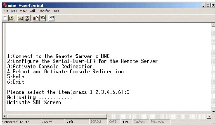
图 3-20. 控制台重定向实例
